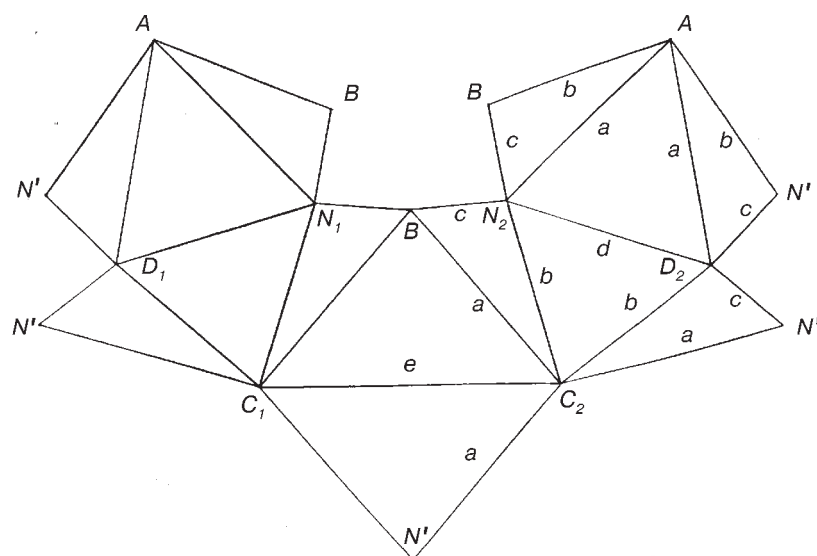
Рис.3. Развертка многогранника Штефена.
